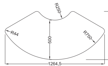
- DIMENSIONI TAVOLO ARCO - Dimension Table Arco - Dimensions Table Arco
